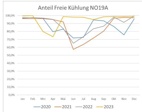
Abbildung 9: Anteil der freien Kühlung 2020 bis 2023
