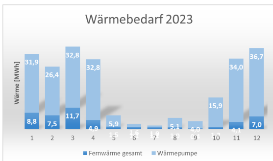
Abbildung 11: Verbrauch an Wärmeenergie 2023
