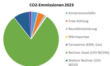
Abbildung 12: Anteile der CO 2 Emissionen aus Elektrizität, Kälte und Wärme im Jahr 2023
