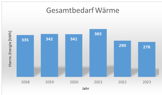
Abbildung 10: Witterungsbereinigter Gesamtwärmeverbrauch in den Jahren 2018 bis 2023
