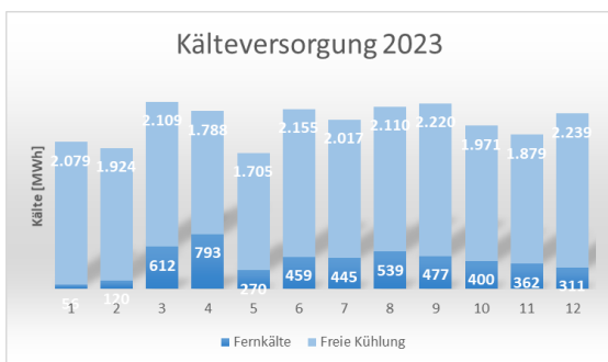
Abbildung 8: Kälteversorgung im Jahr 2023
