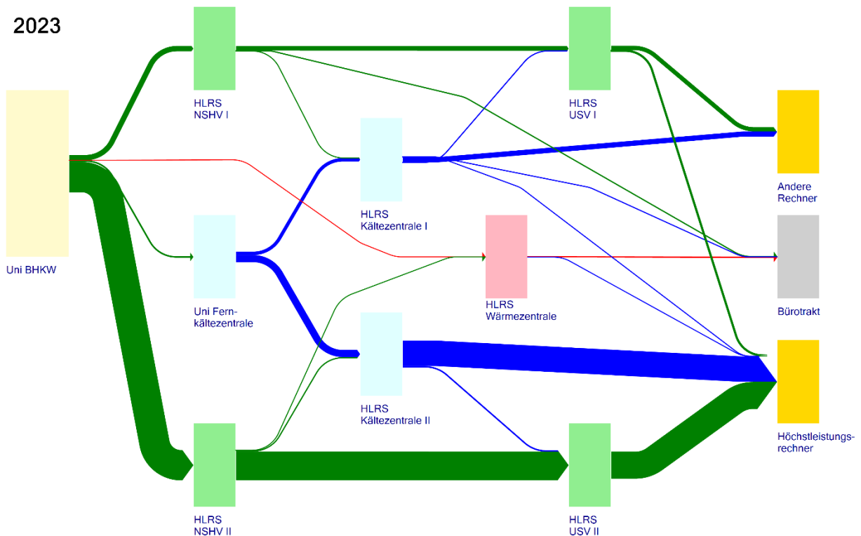
Abbildung 5 Vereinfachtes Energiefluss-Schema des HLRS
